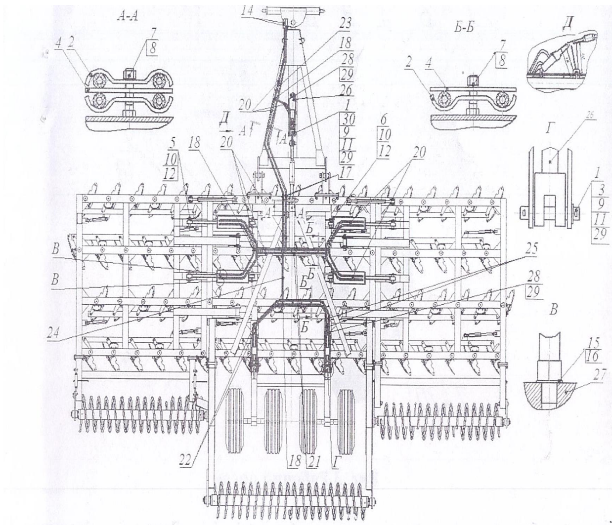
Рис. 2 — Гидротрасса БДМ- 8х4П складная
