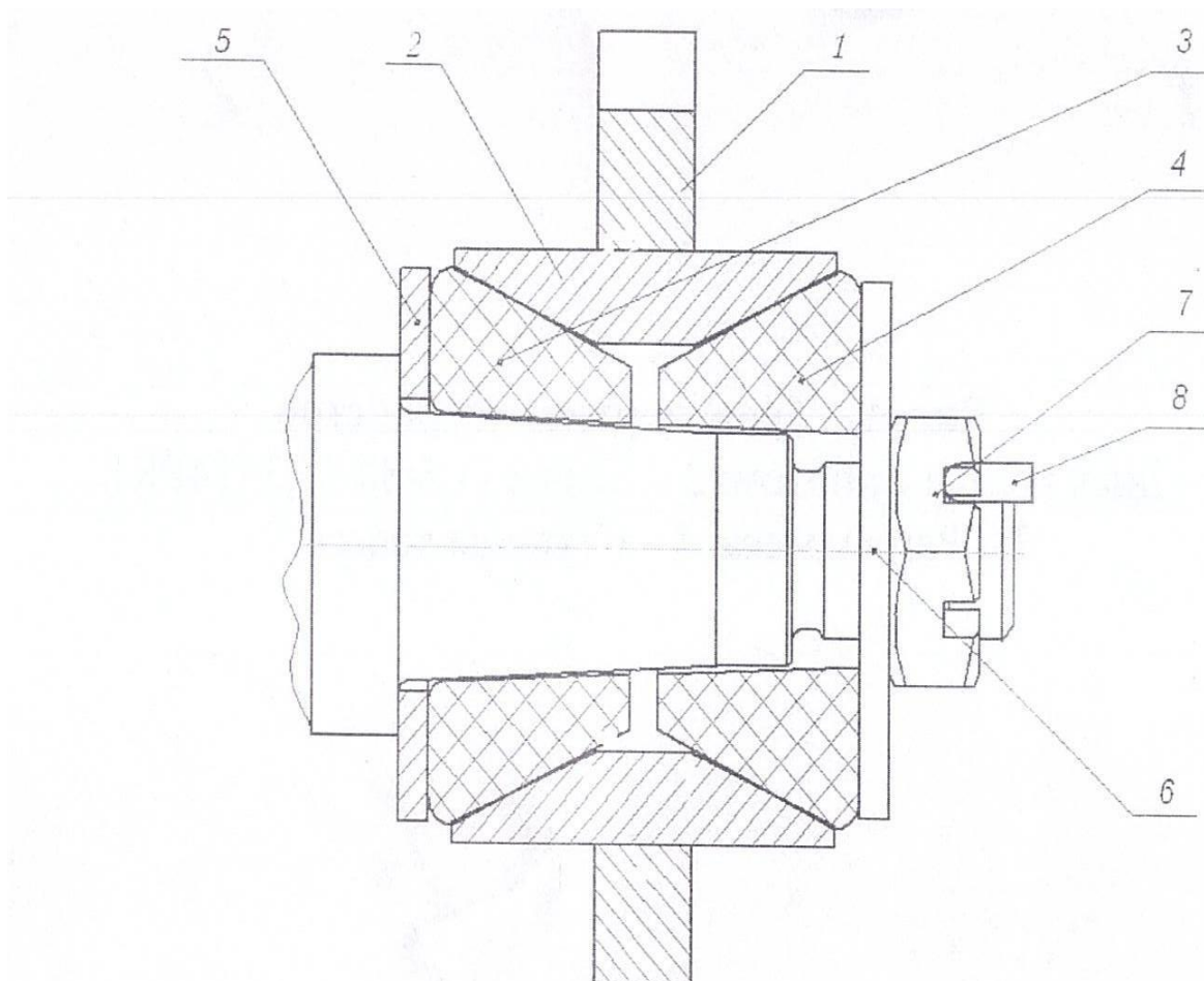
Рис. 6 - Соединение секции шлейф-катка с кронштейном
