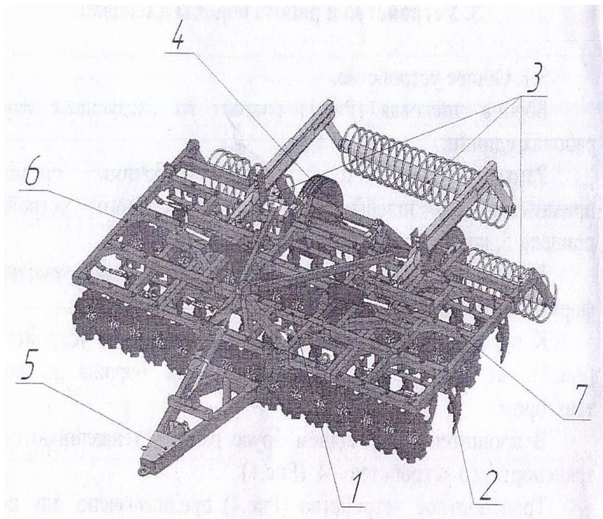
Рис. 1. – Борона дисковая модульная БДМ-8х4П складная
