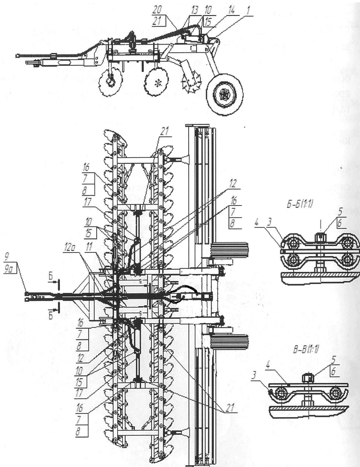
Рис. 2 Гидротрасса БДМ-5х2П(скл.)
