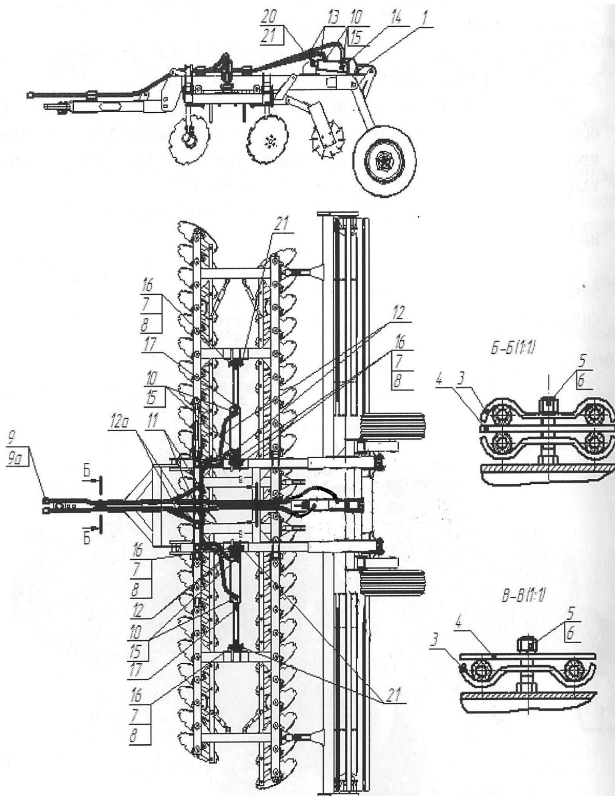
Рис. 2 Гидротрасса БДМ-6х2П
