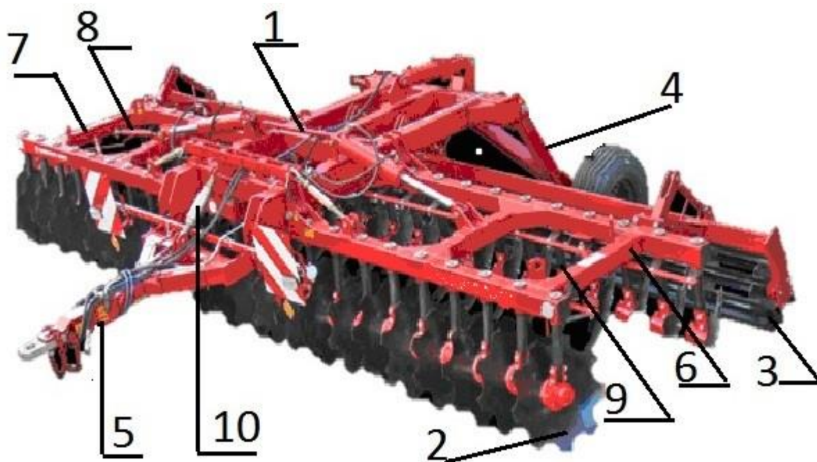
Рис.1 Боро́на дисковая прицепная БДМ-6х2П
